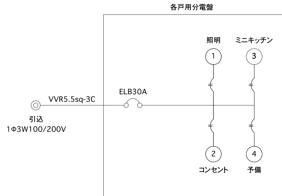
盤結線図
